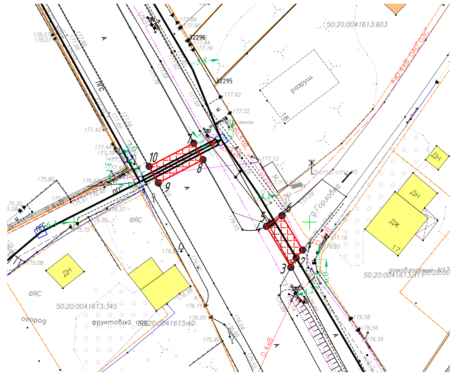
План М 1:500 Система координат МСК -50 зона
