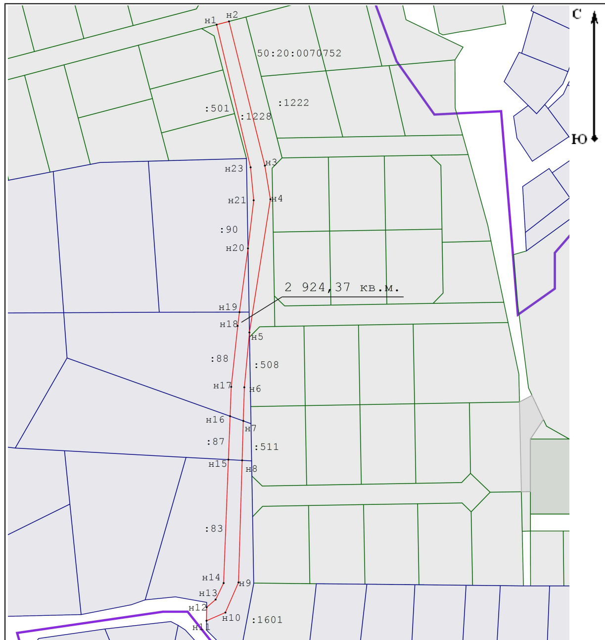
Чертеж № 1
