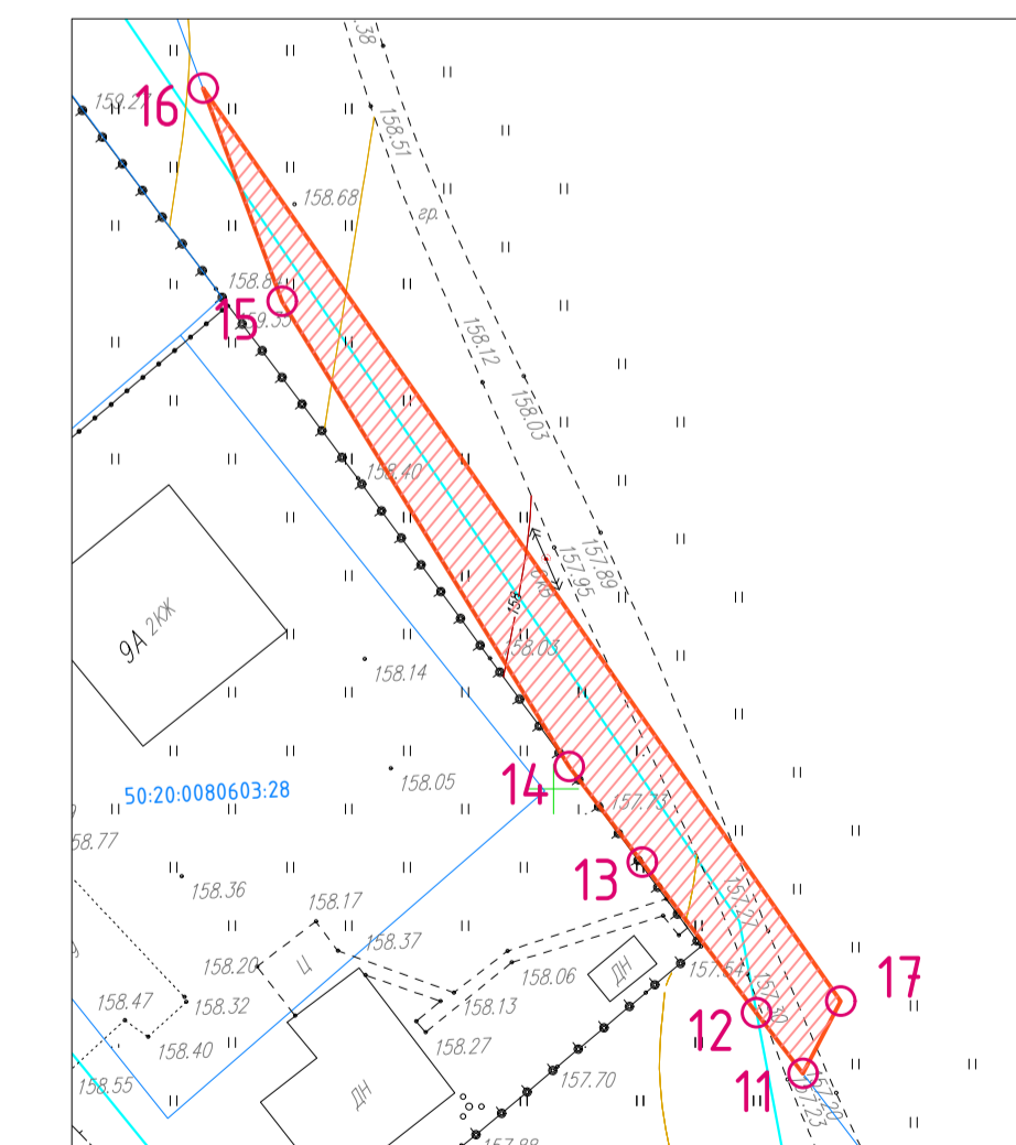
Чертеж границ части (283:чз2) земельного участка с кадастровым номером: 50:20:0080607:283, относительно которого заключается договор аренды М 1:500
