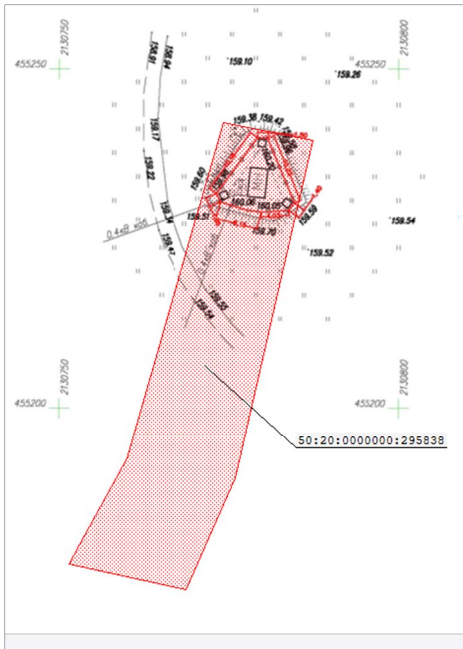
Рисунок 4 – Планировочные ограничения
