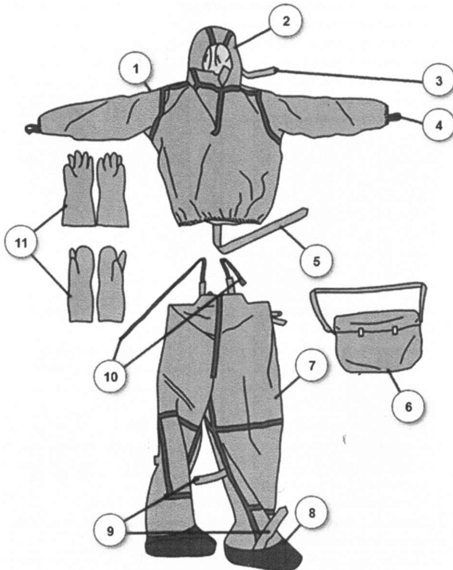
Рис. 46. Костюм легкий защитный /1-1.
