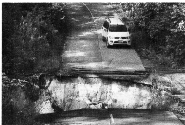
Рис. 2. Карстовая просадка (провал) земной поверхности
