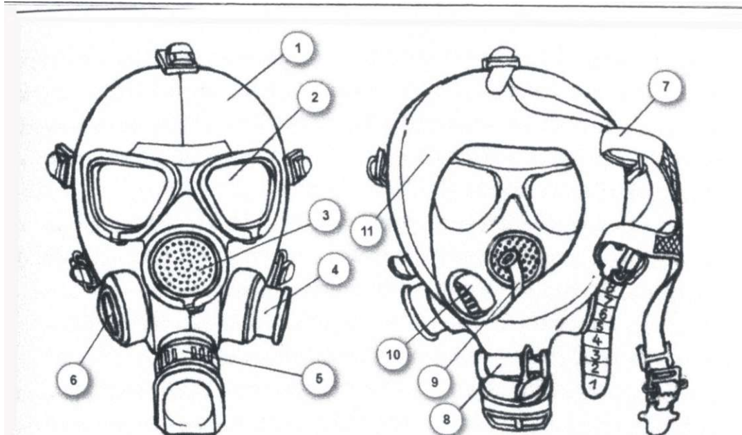
Рис. 26. Устройство гражданского противогаса ГП-9.
