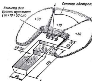
Окопы для стрельбы лежа: а – из автомата; б – из пулемета Окопы для ведения флангового огня должны иметь бруствер со стороны противника высотой 30 см на всю длину окопа
